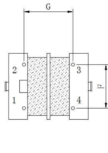
底视图
