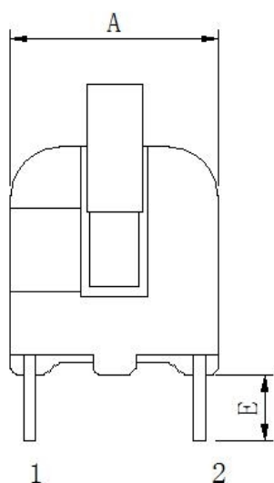
主视图
